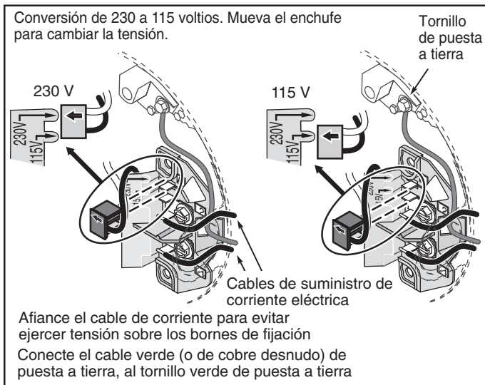
Figura 5: Conexión de los cables del motor, Enchufe.
